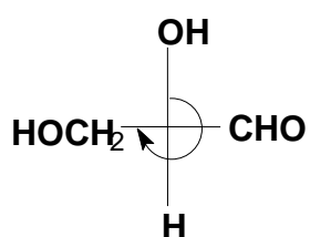
( R )-Глицериновый альдегид
