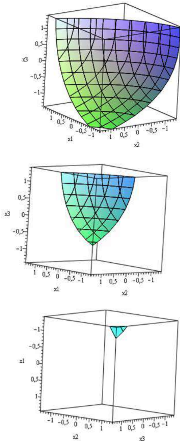
Рис. 7. Метод динамического расслоения
