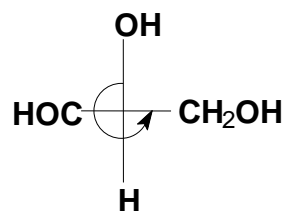
( S )-Глицериновый альдегид
