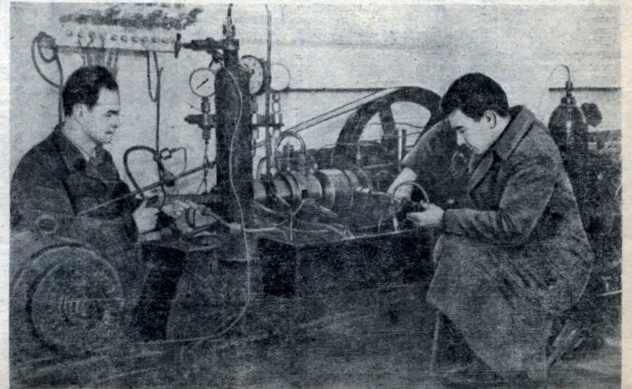
На снимке: студенты В. Гочев и С. Георгиев за сборкой компрессора высокого давления.
